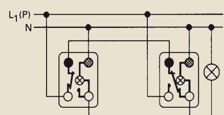
Wechselschalter
