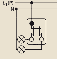
Serienschalter
