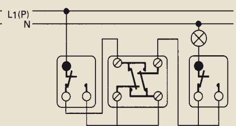
Wechselschalter
