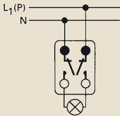
Ausschalter, 2-polig
