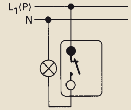
Ausschalter, 1-polig
