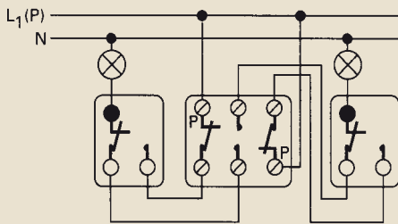
Wechselschalter
