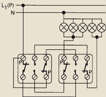
Doppelwechselschalter
