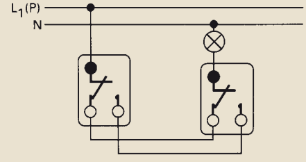
Wechselschalter Wechselschalter
