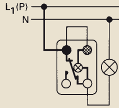
Universalschalter als Ausschalter, beleuchtet
